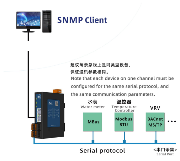
场景2: 集成串口协议到SNMP Client
