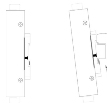
导轨式安装
