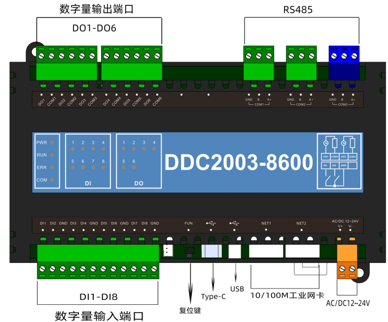
图一 电源和通讯示意图
