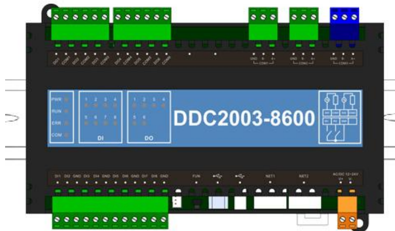
图五 导轨式
