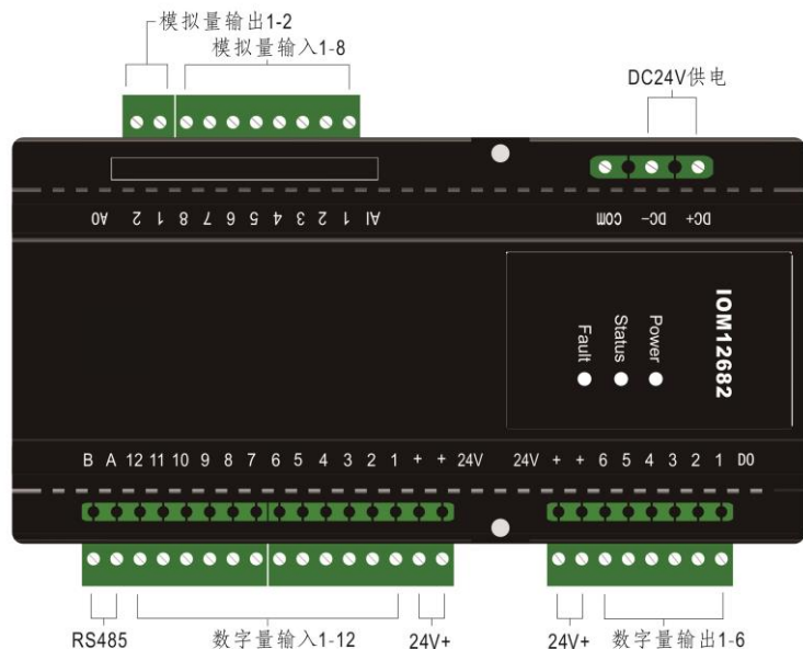
图 1 电源和通讯示意图 规格: 174mm*108mm*58mm 重量: 300g 导轨式安装
