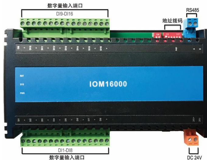
图一 数字量输入接线示意图
