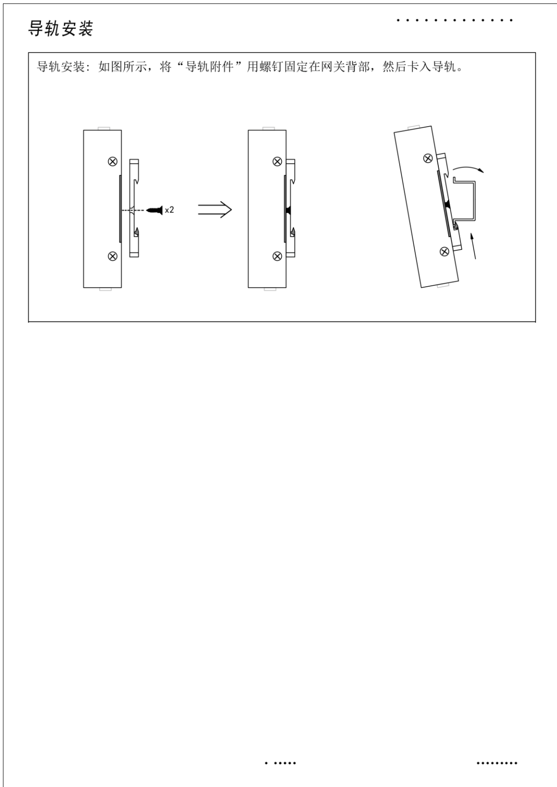
图 17-3 MOD2004-A9 安装图
