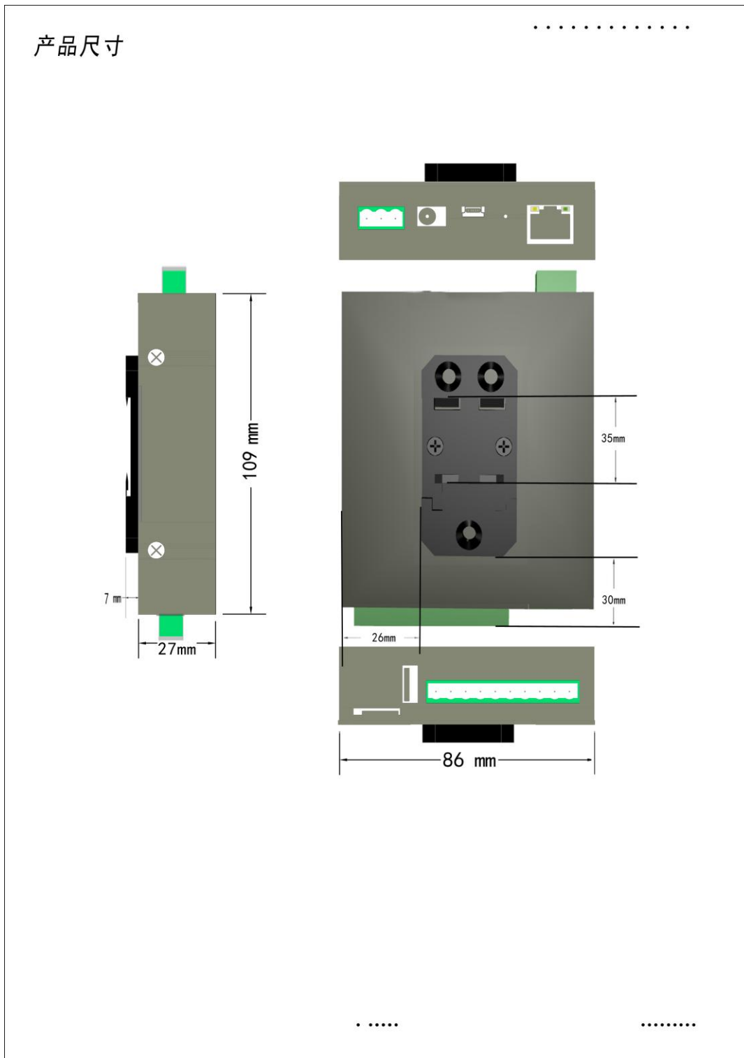
图 16-1 MOD1002-ARM 产品尺寸图
