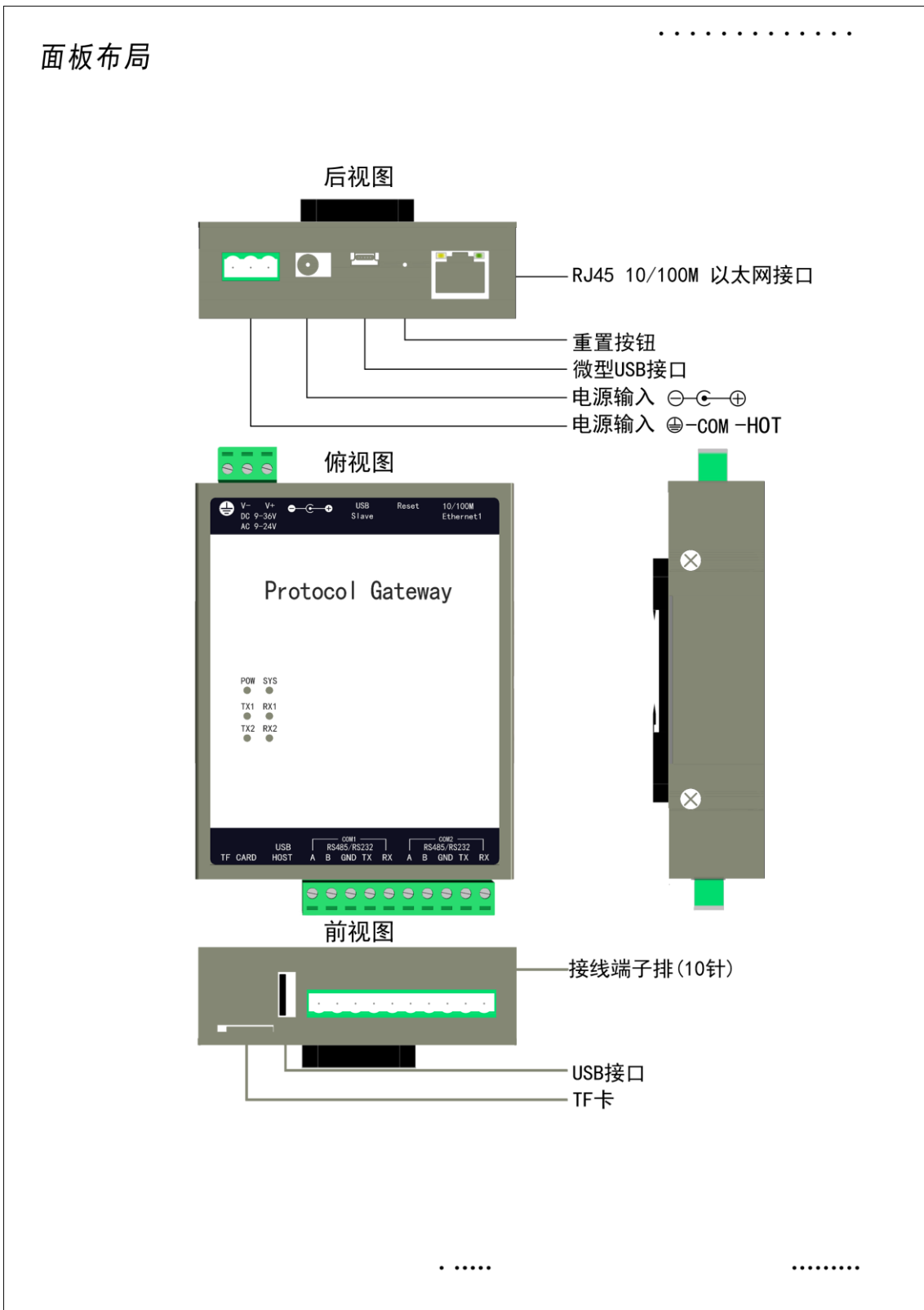
图 16-2 MOD1002-ARM 面板布局图
