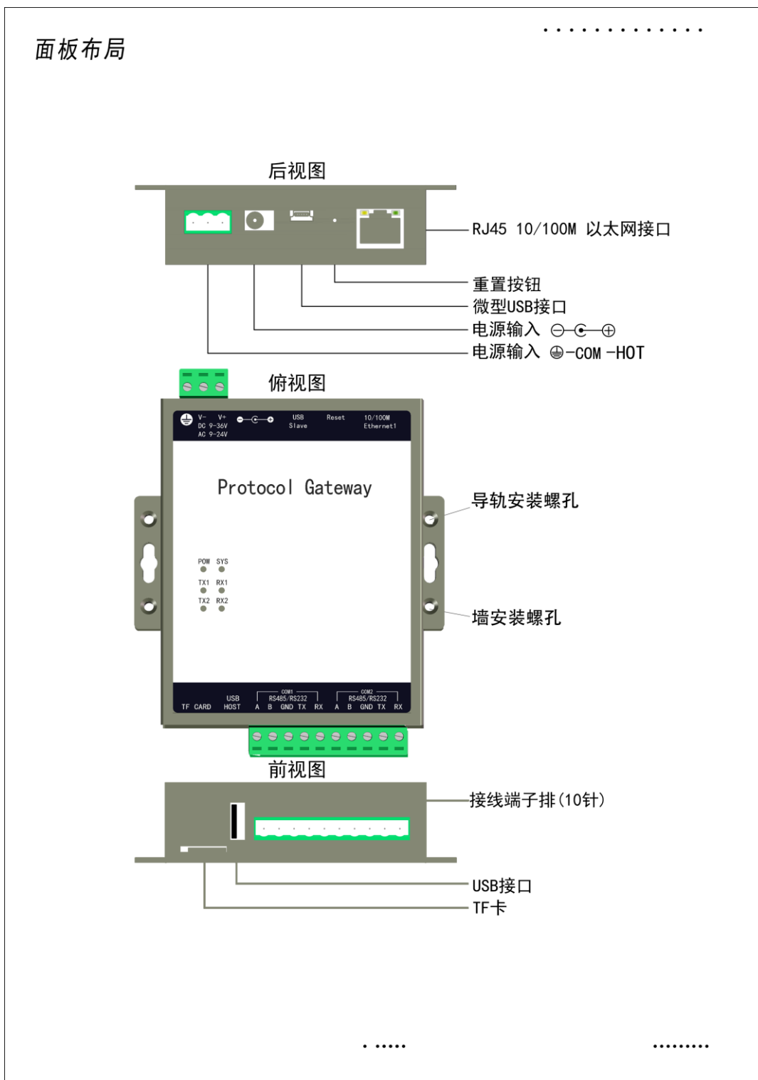
图 18-2 MOD1002-ARM-B 面板布局图
