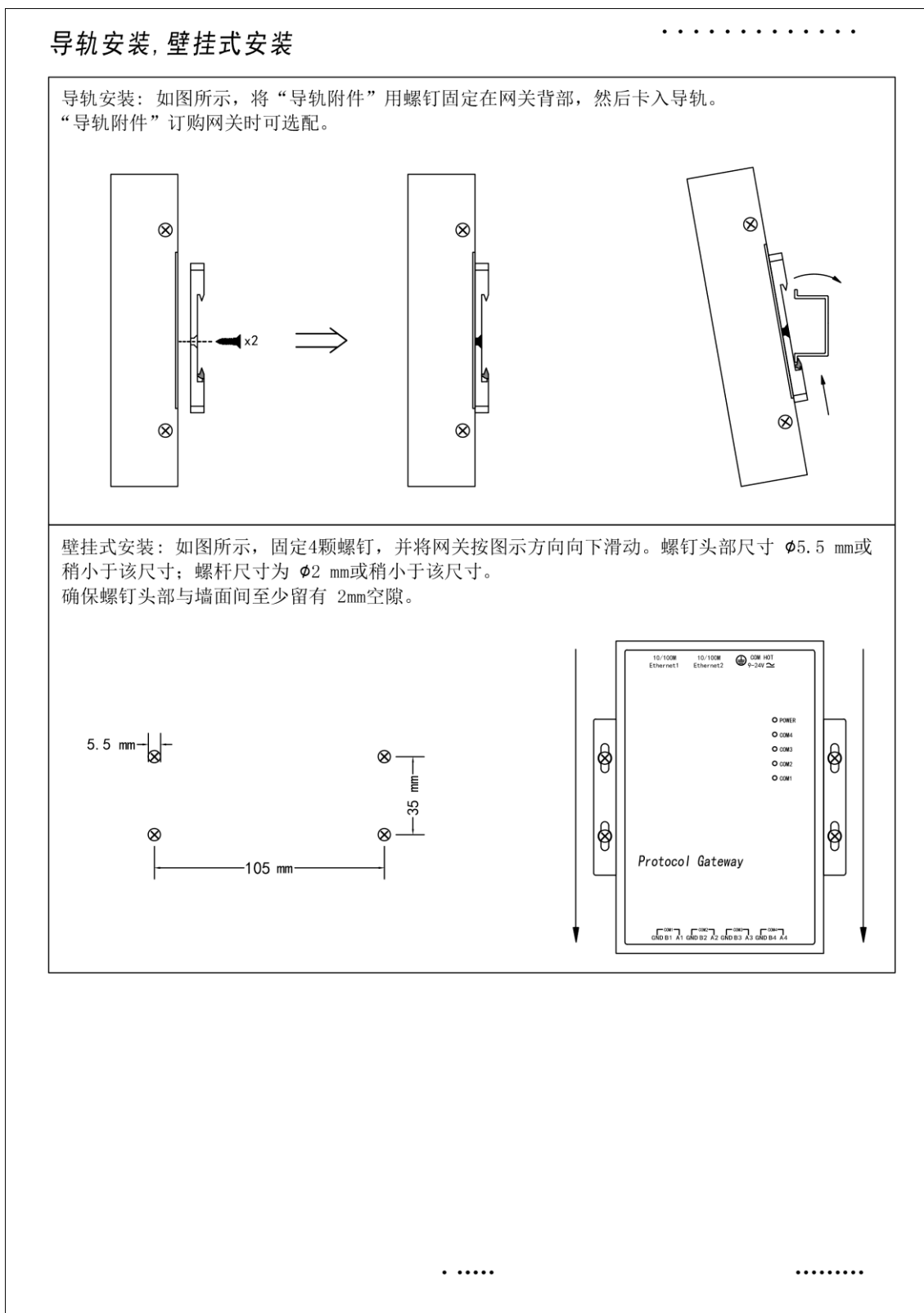
图 15-3 MOD2004-ARM 安装图
