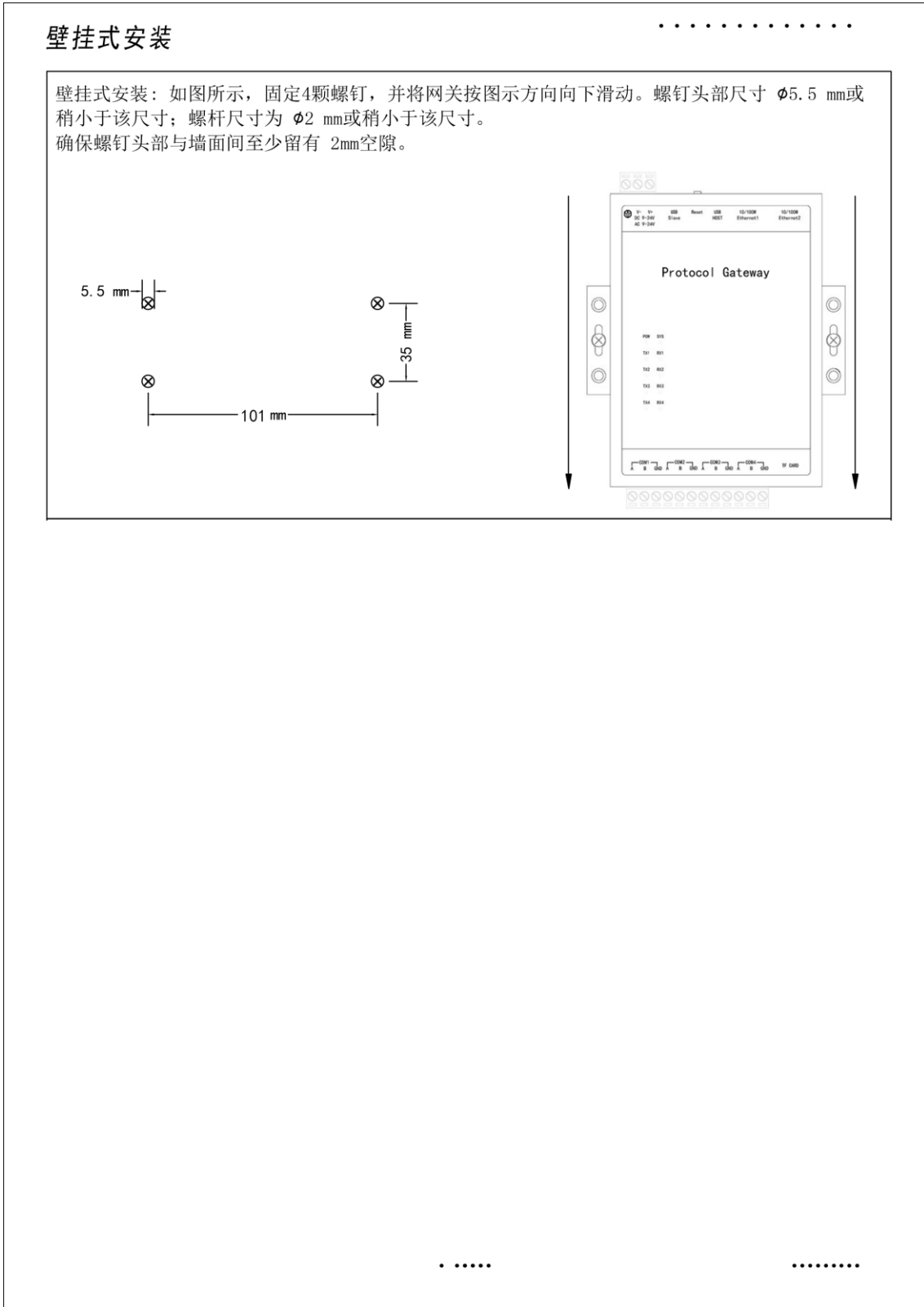
图 19-3 MOD2004-A9-B 安装图
