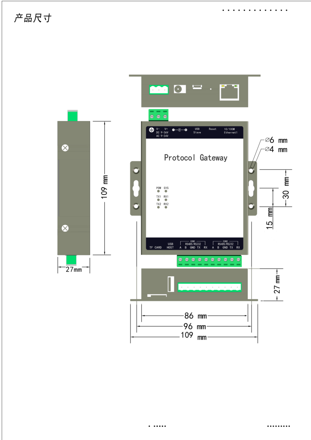
图 18-1 MOD1002-ARM-B 产品尺寸图
