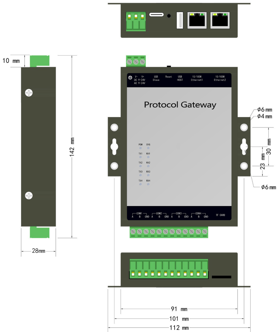
图 19-1 MOD2004-A9-B 产品尺寸图
