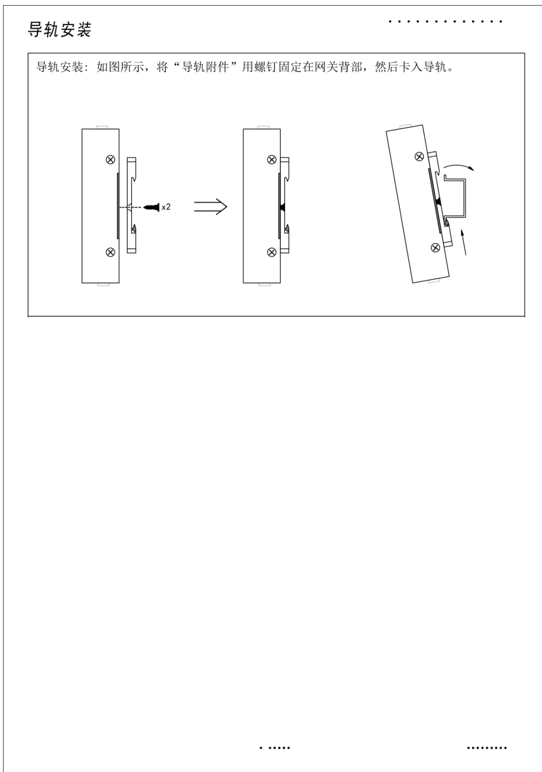
图 16-3 MOD1002-ARM 安装图
