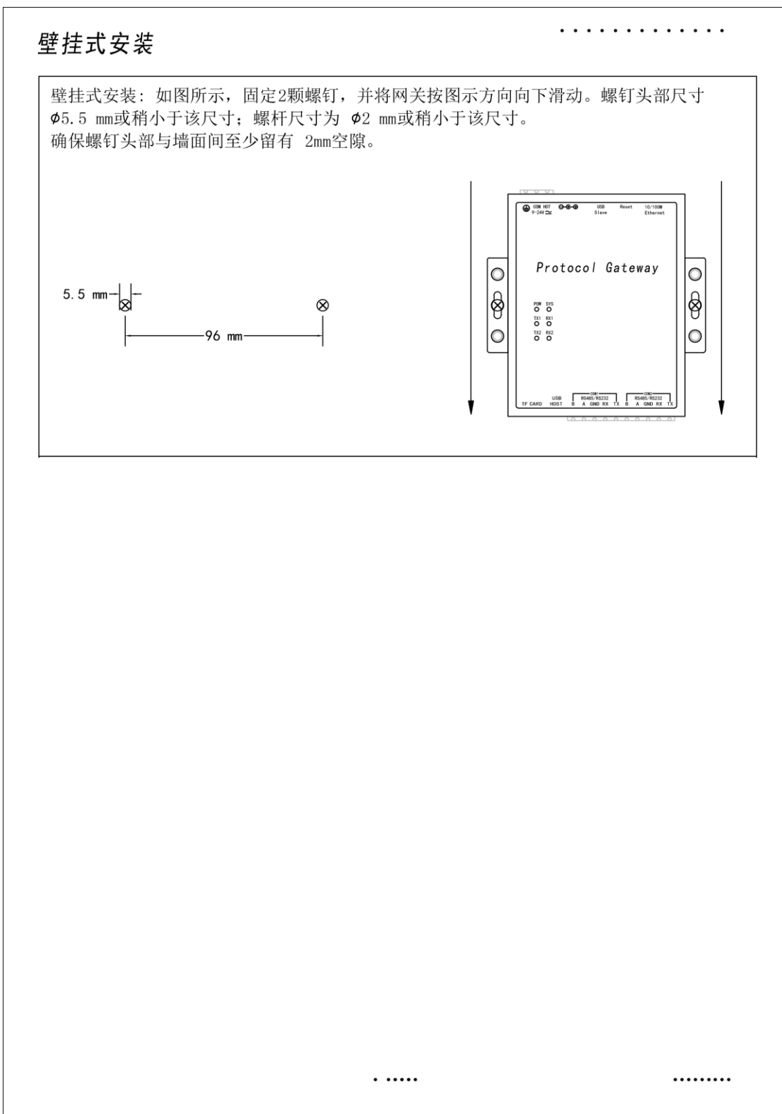
图 18-3 MOD1002-ARM-B 安装图
