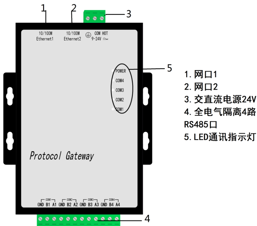
图 6-1 网关接口示意图
