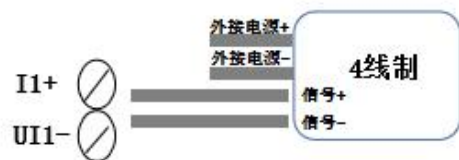
图四 模拟量输入接线示意图
