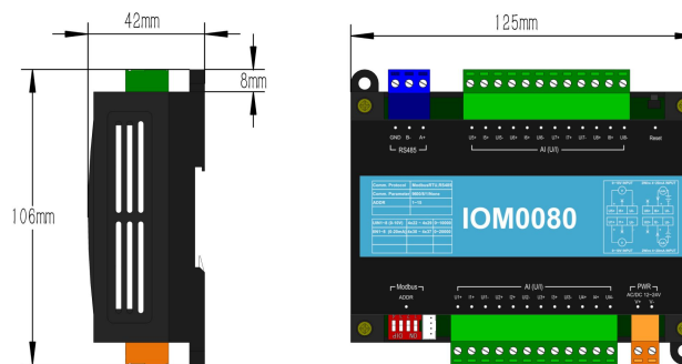
图六产品尺寸125mm*106mm*42mm (LxWxH) 重量200g
