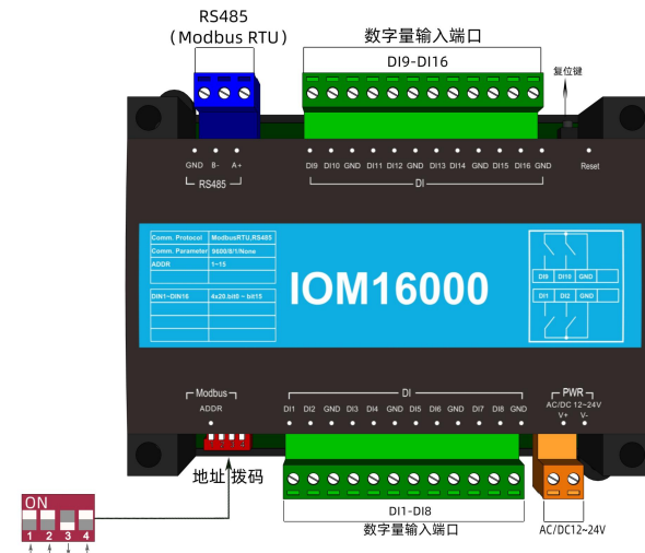
图一 数字量输入接线示意图 (以第一通道为例)
