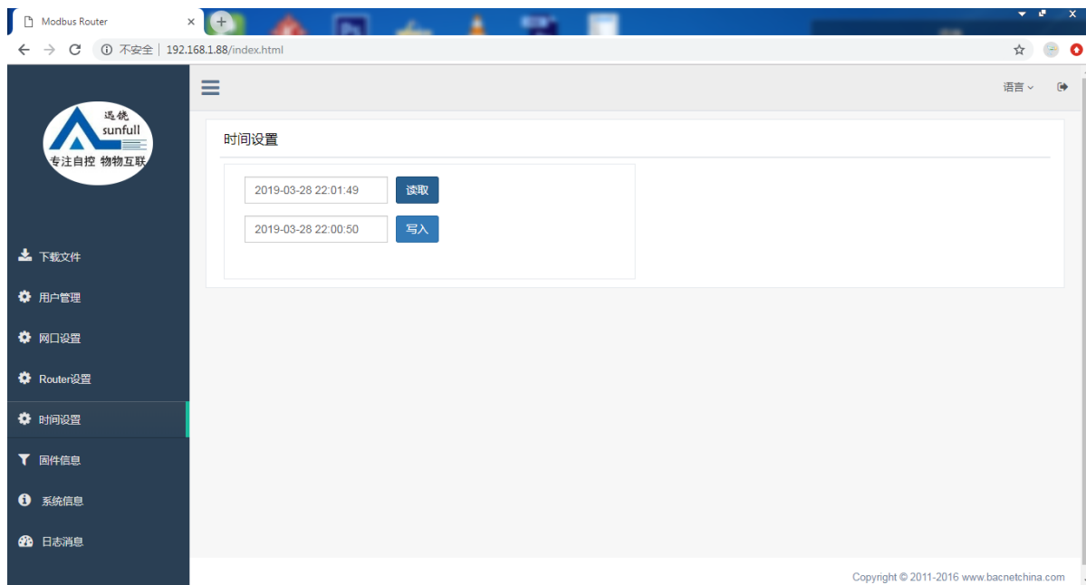
图 3-6-1 时间设置
