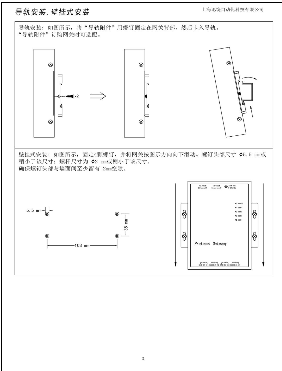
图 9-3 HUB2004 安装图
