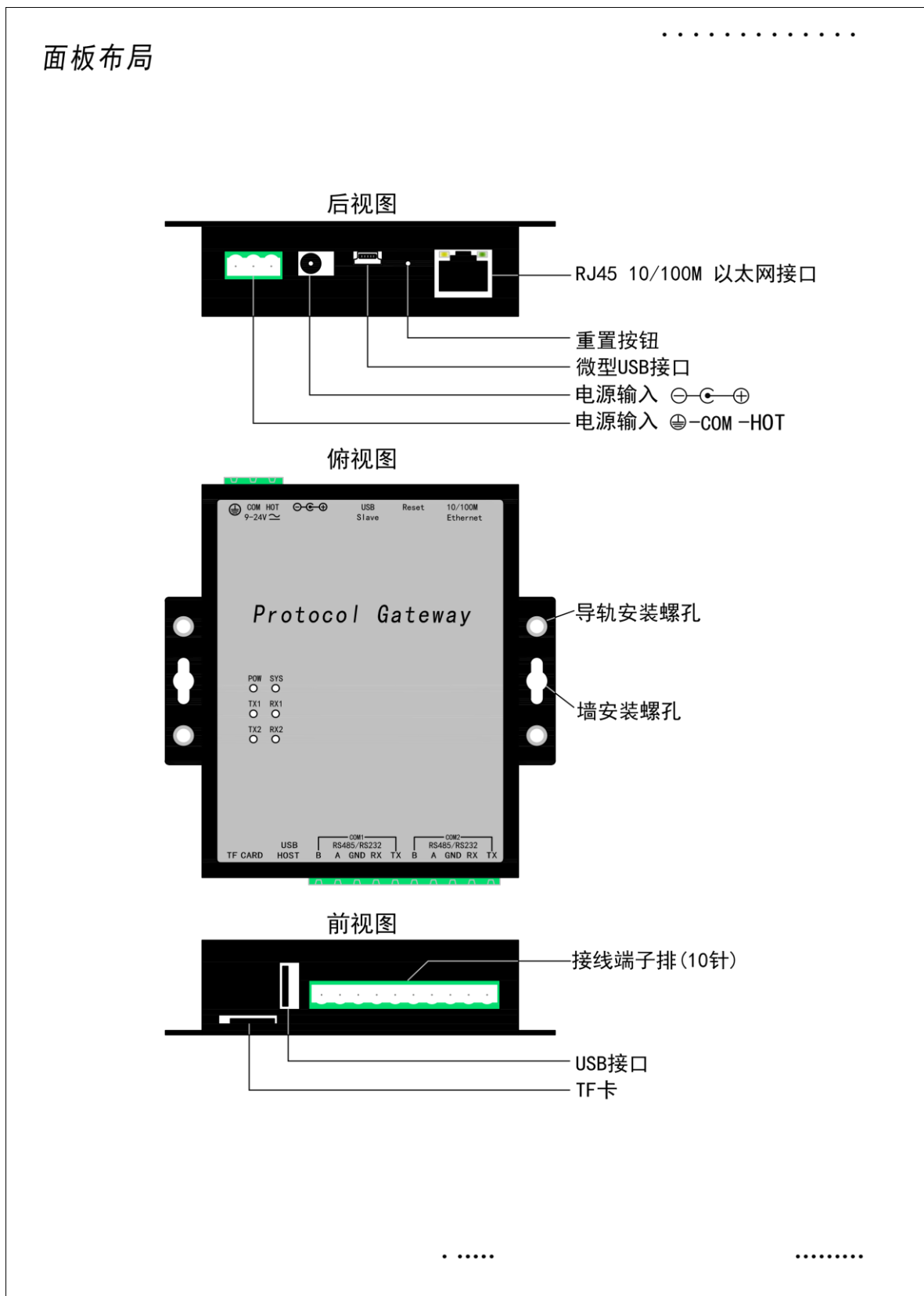
图 10-2 HUB1002 面板布局图
