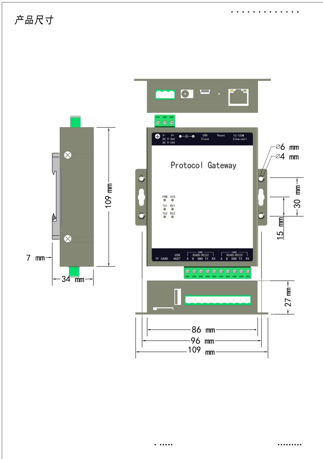
图 10-1 HUB1002 产品尺寸图
