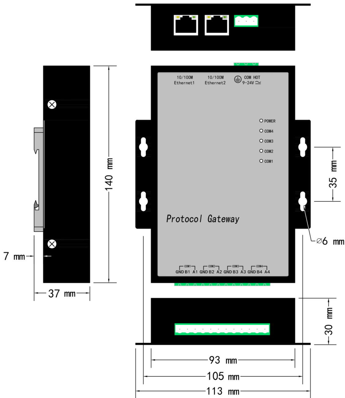
图 9-1 HUB2004 产品尺寸图
