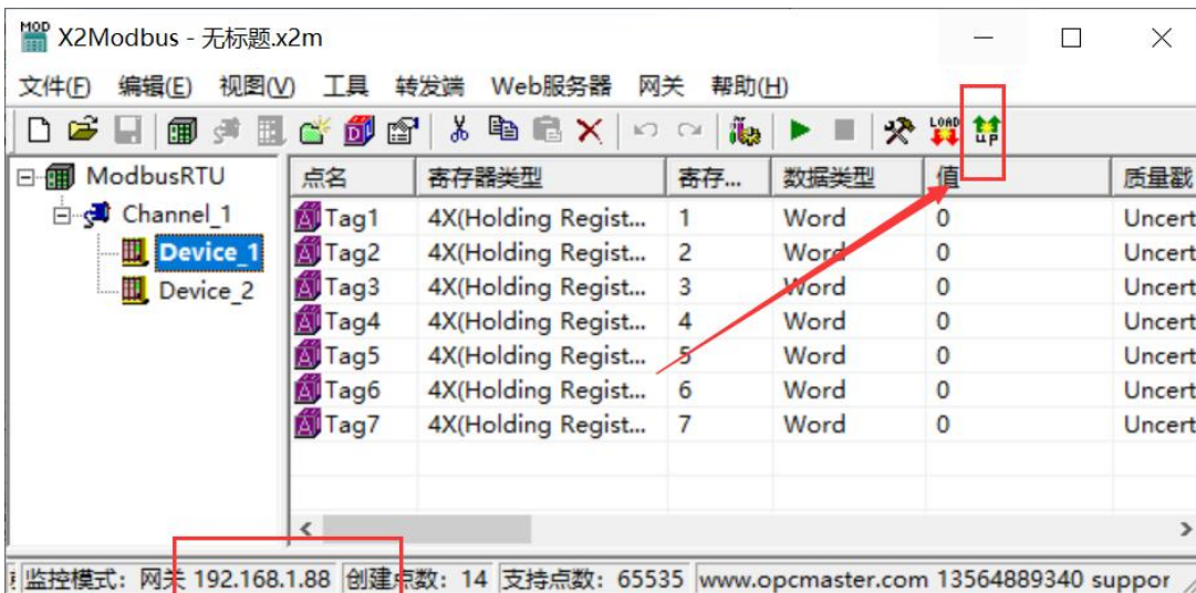
图 3-9-2 选择上传工程
