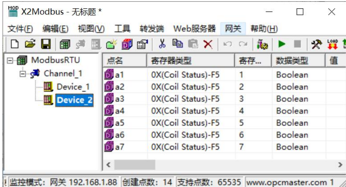
图 3-6-15 导入 EXCEL 表完成
