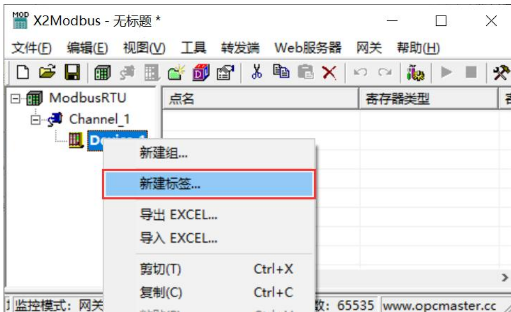
图 3-6-1 选择新建标签
