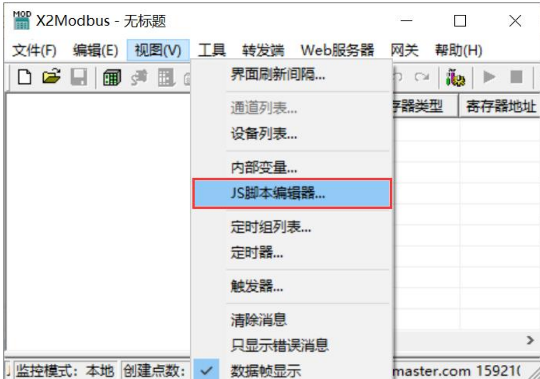
图 6-1-1 打开 JS 脚本编辑器
