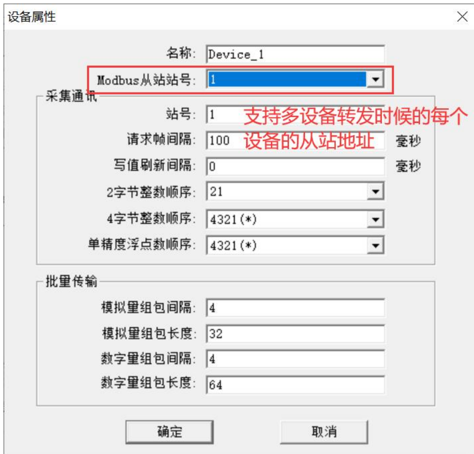
图 3-7-3 Modbus 多设备从站地址
