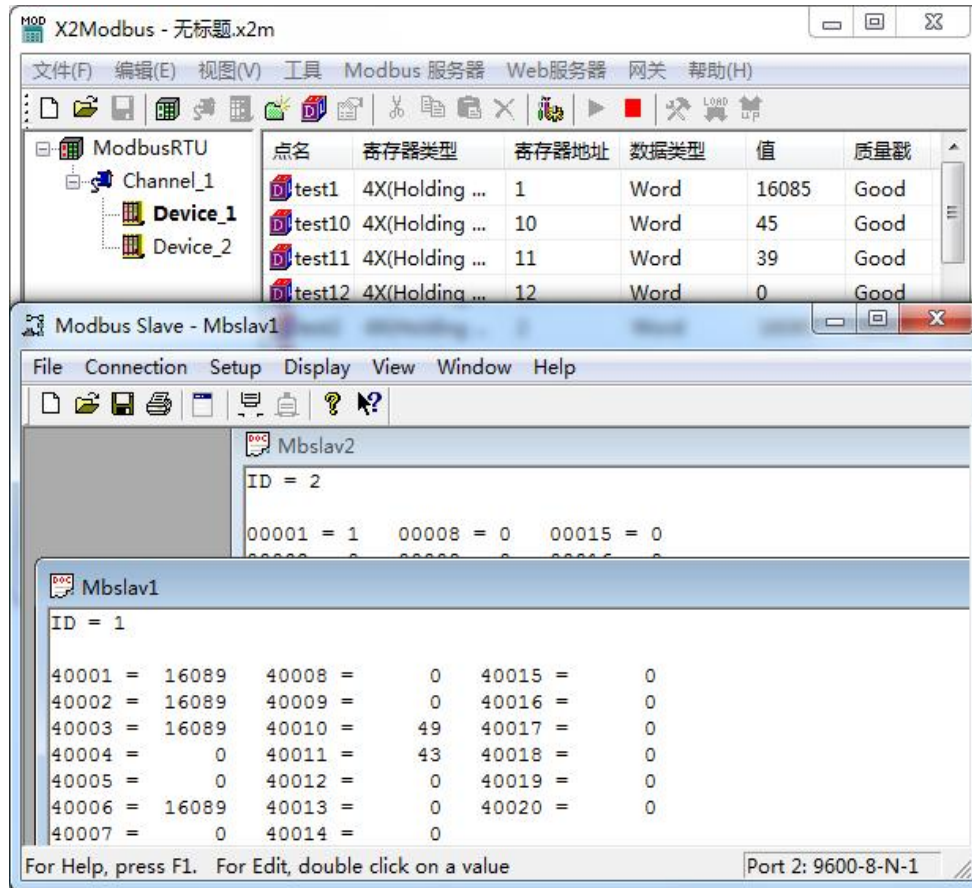
图 3-8-4 采集数据成功
