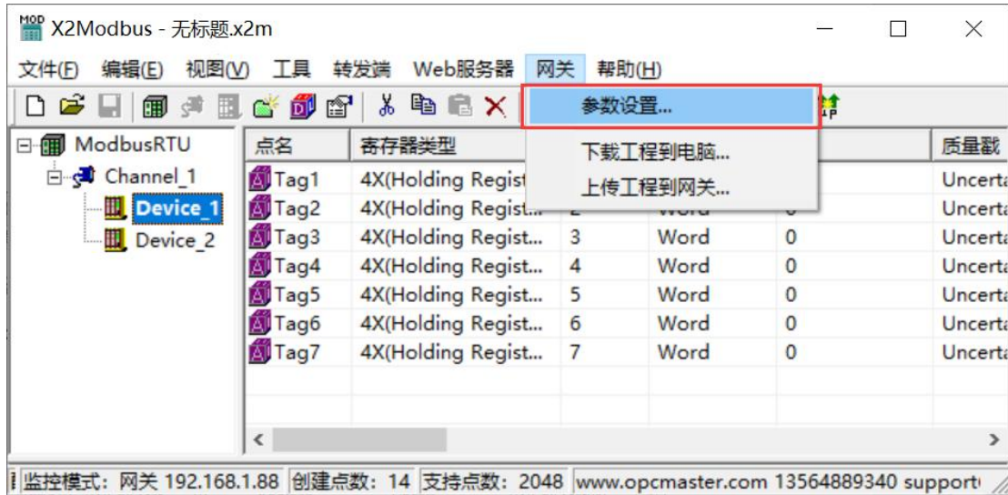
图 3-10-1 选择网关参数设置
