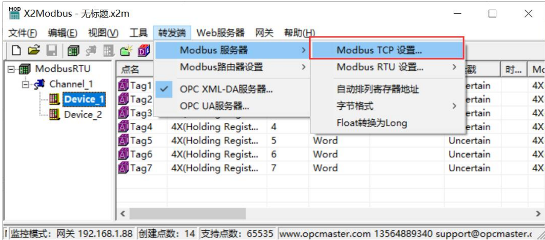
图 3-7-1 选择 ModbusTCP 设置
