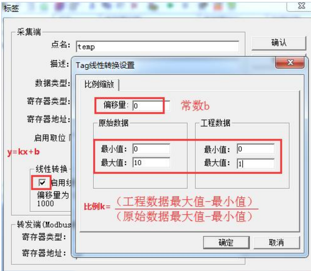
图 3-6-4 线性转换功能
