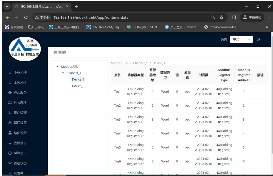
图 4-9-1 查看实时数据
