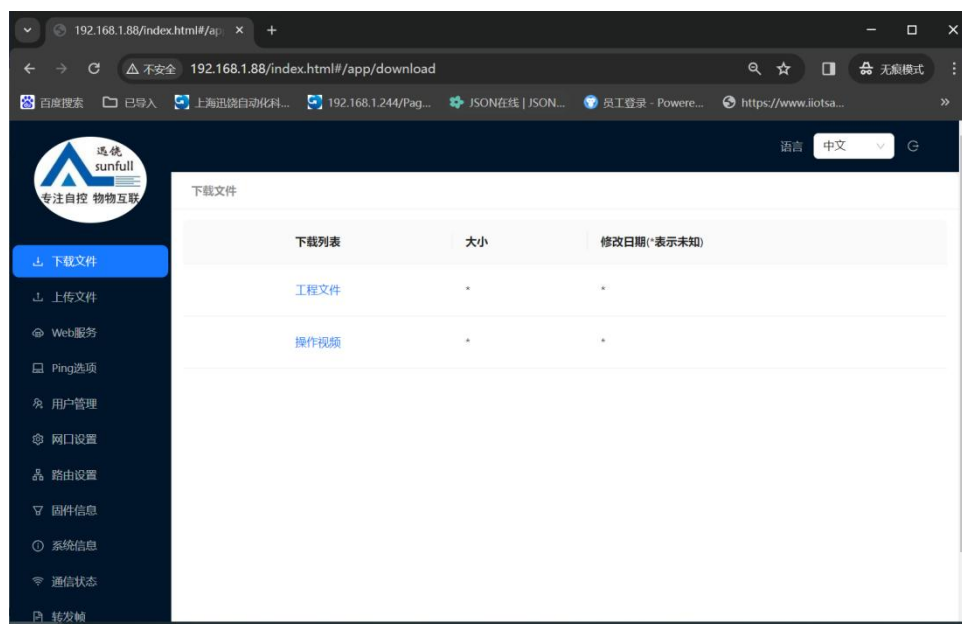
图 4-2-1 下载文件
