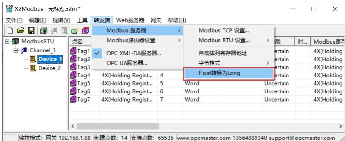
图 3-7-9 Float 转 Long
