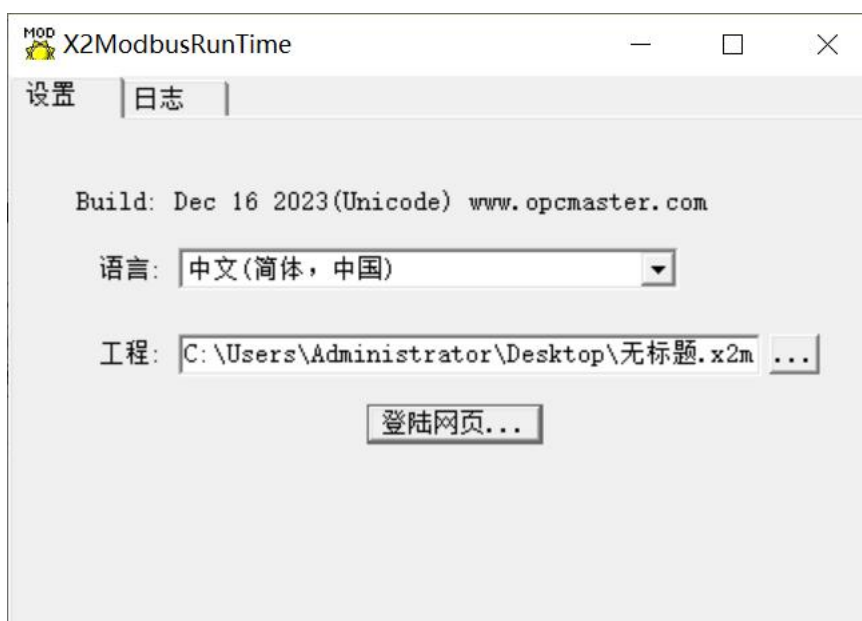
图 3-8-2 X2ModbusRunTime 主界面
