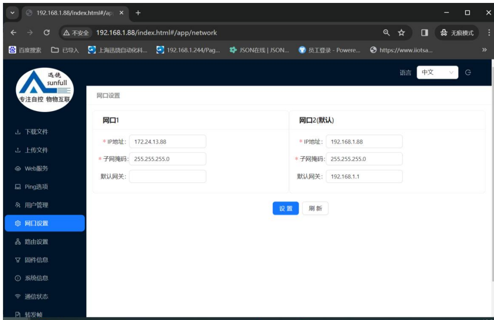
图 4-4-1 网口设置
