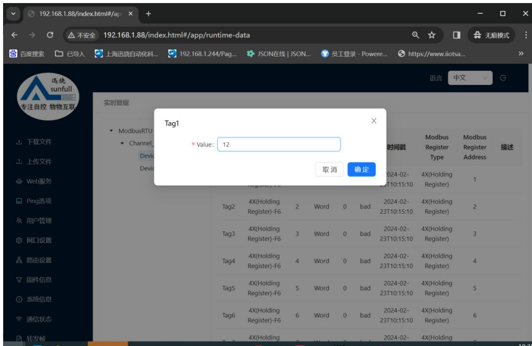
图 4-9-2 写值操作
