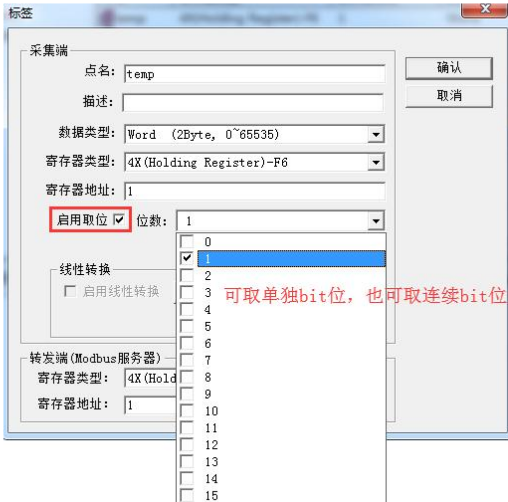
图 3-6-3 取位功能
