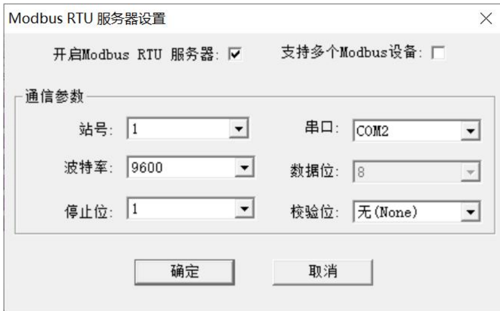
图 3-7-5 RTU 方式参数设定
