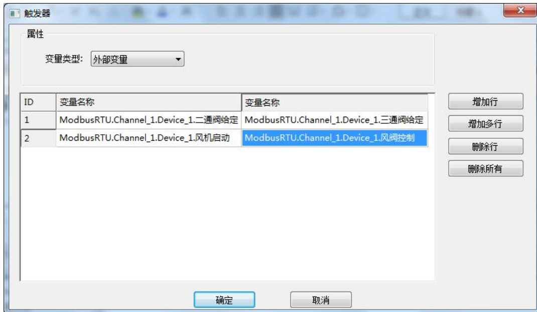
图 3-14-2 触发器编辑窗口
