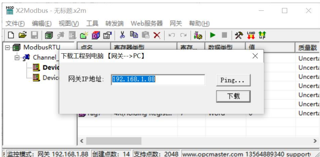
图 3-11-2 下载工程
