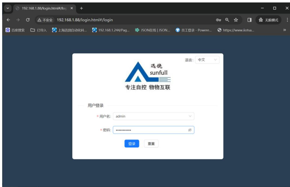
图 4-1-2 用户登录
