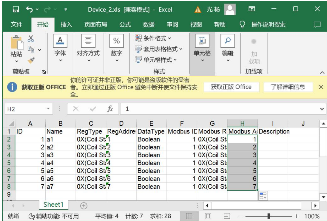
图 3-6-13 编辑 EXCEL 表
