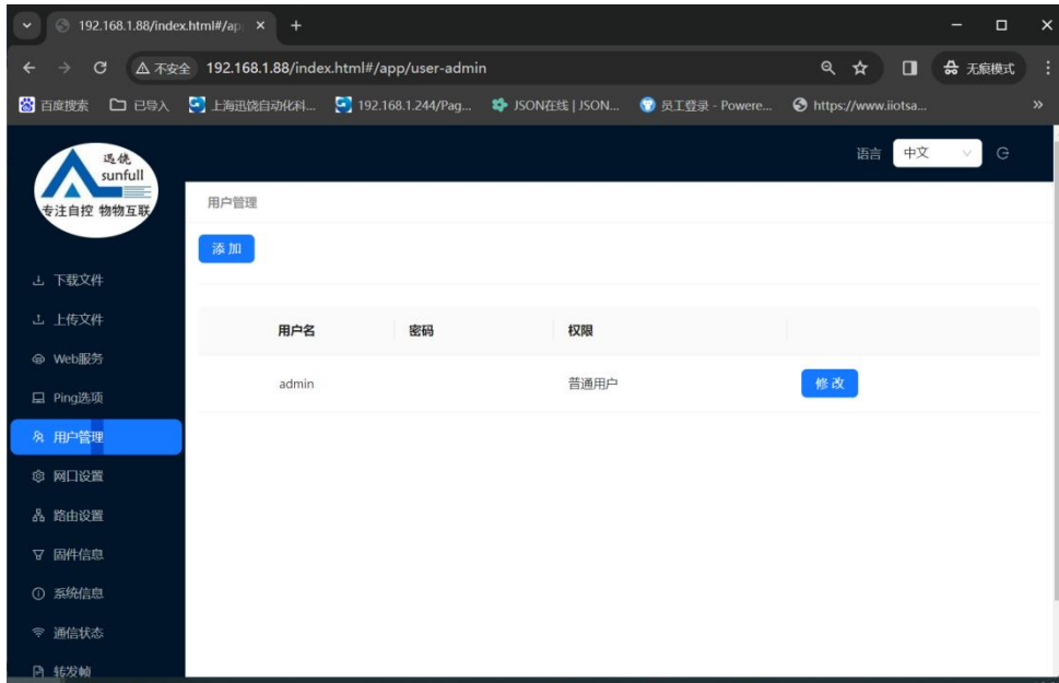
图 4-3-1 用户管理
