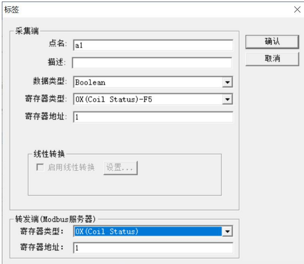
图 3-6-9 新建标签
