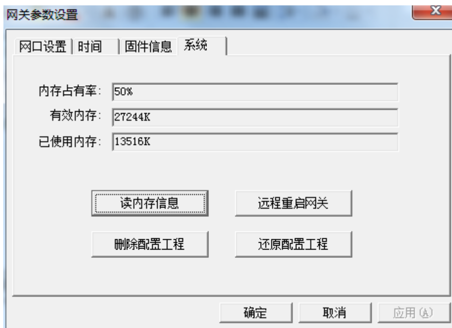
图 3-10-6 系统设置
