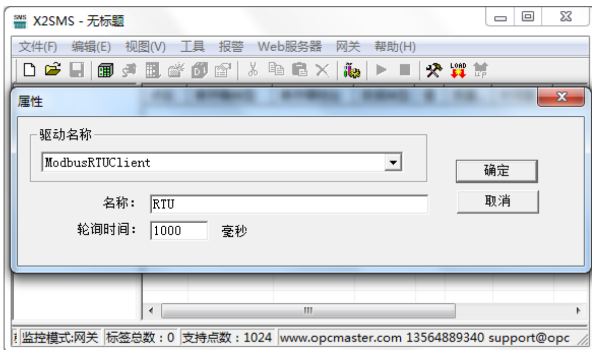
图 3-3-3 驱动属性
