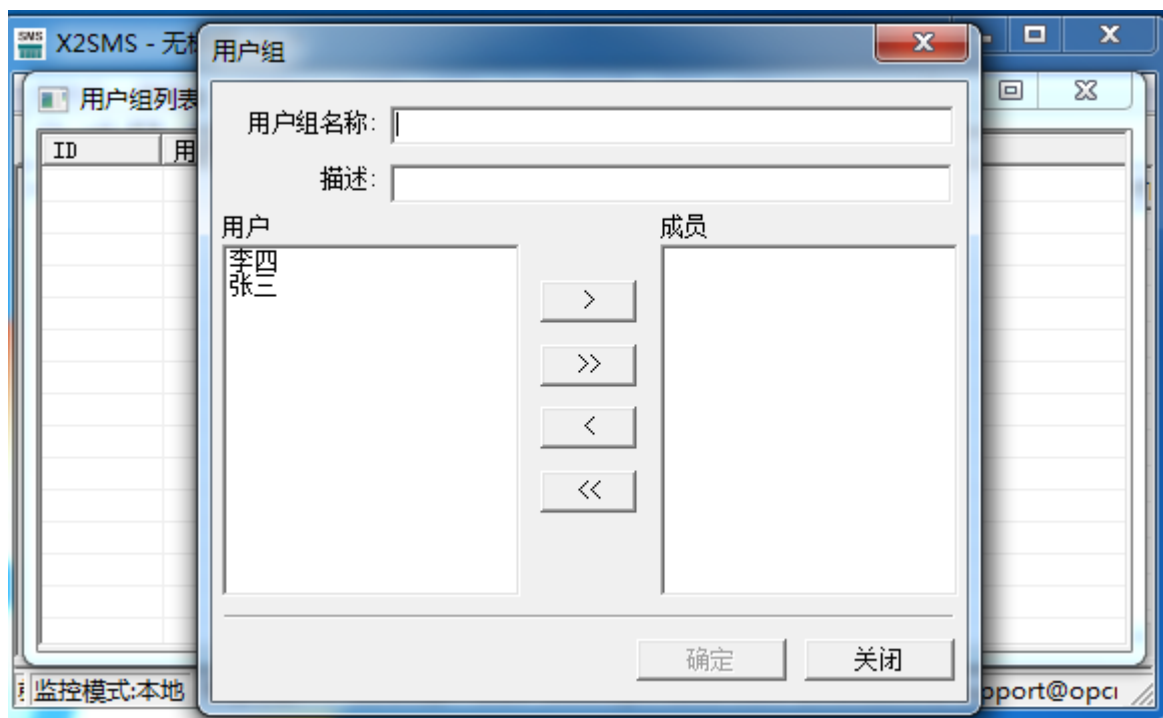
图 3-7-7 新建分组
