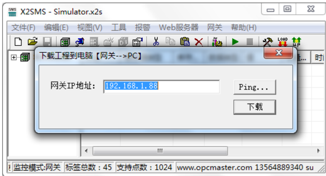
图 3-11-2 下载工程
