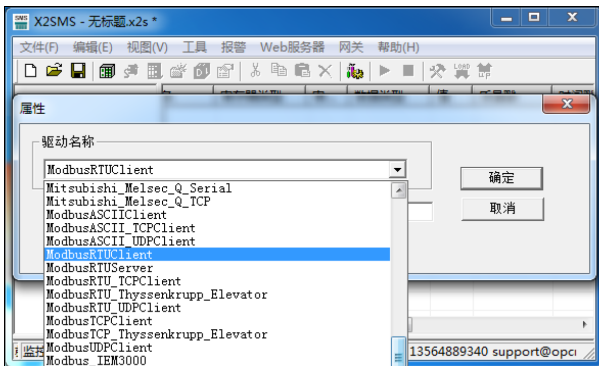
图 3-3-2 选择驱动
