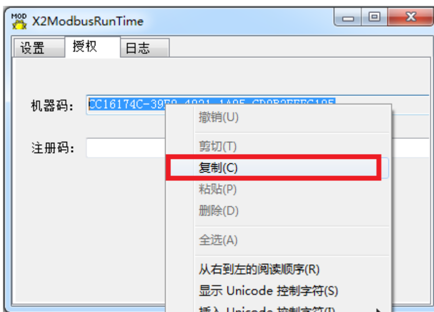
图 3-12-2 复制机器码
