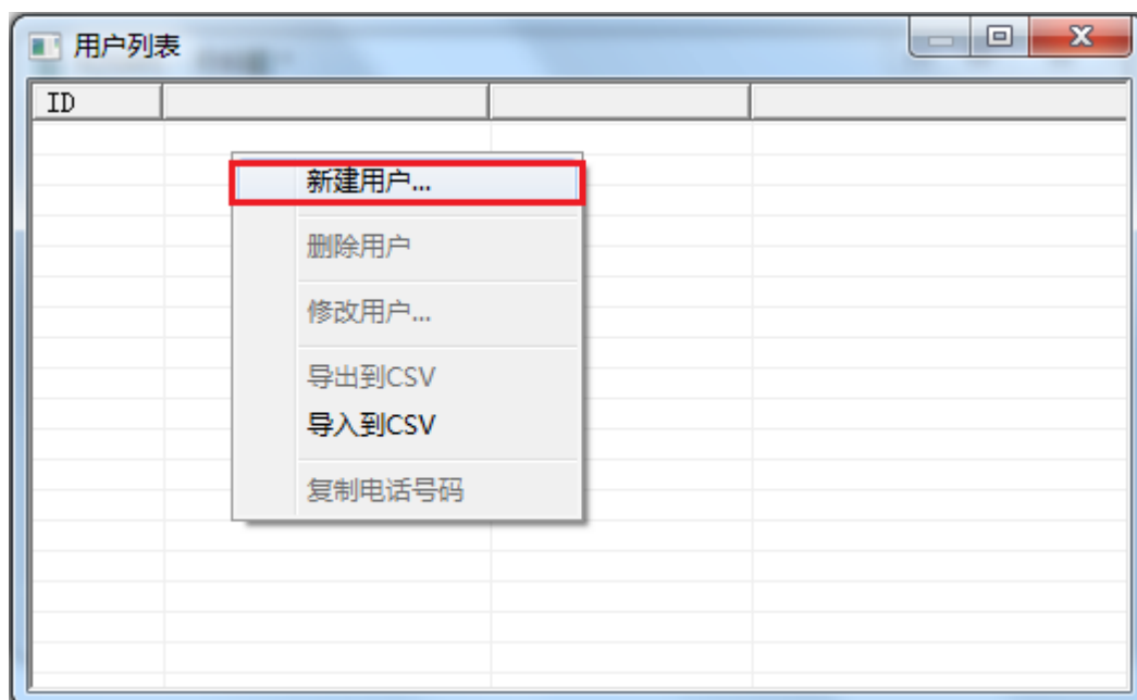
图 3-7-2 新建用户
