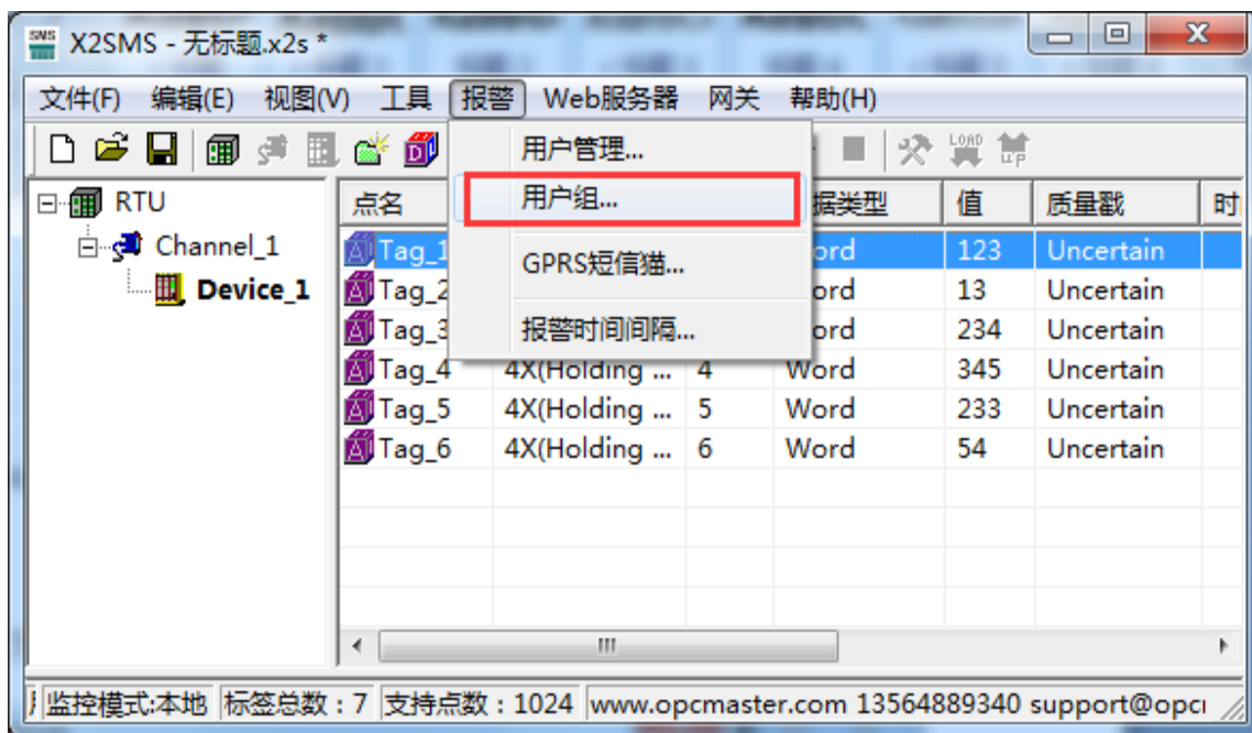
图 3-7-5 选择用户组
