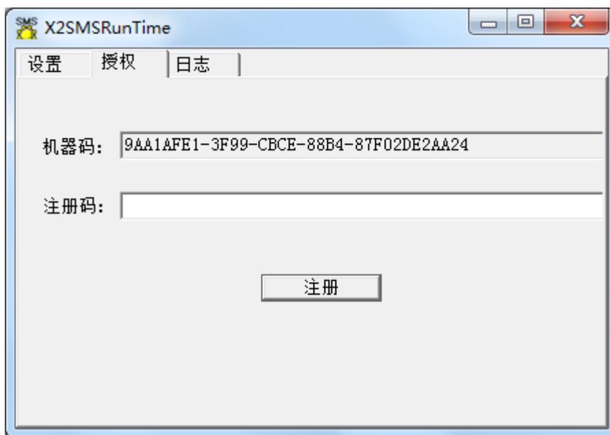
图 3-12-1 产生机器码
