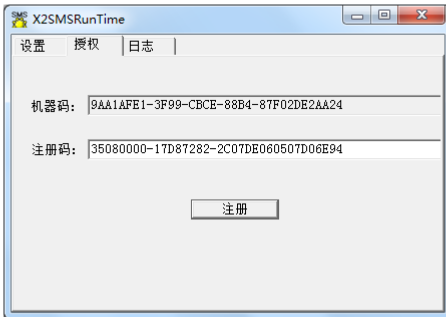
图 3-12-3 完成注册
