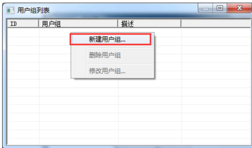
图 3-7-6 新建用户组
