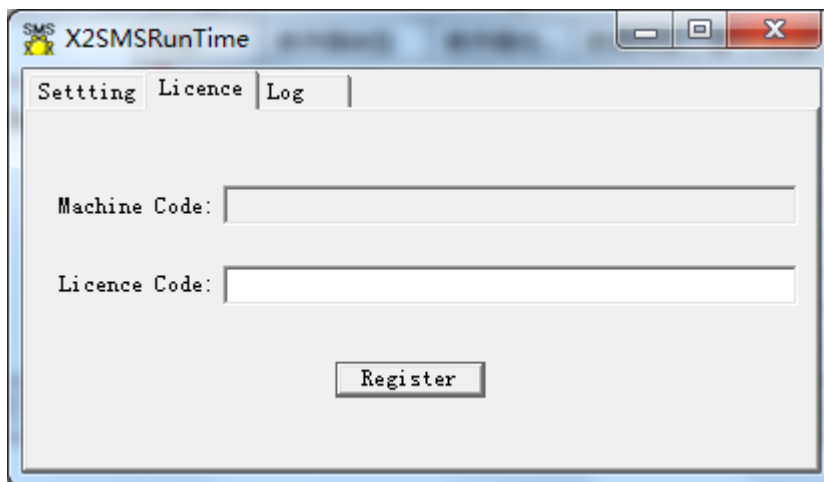
图 3-8-3 软授权
