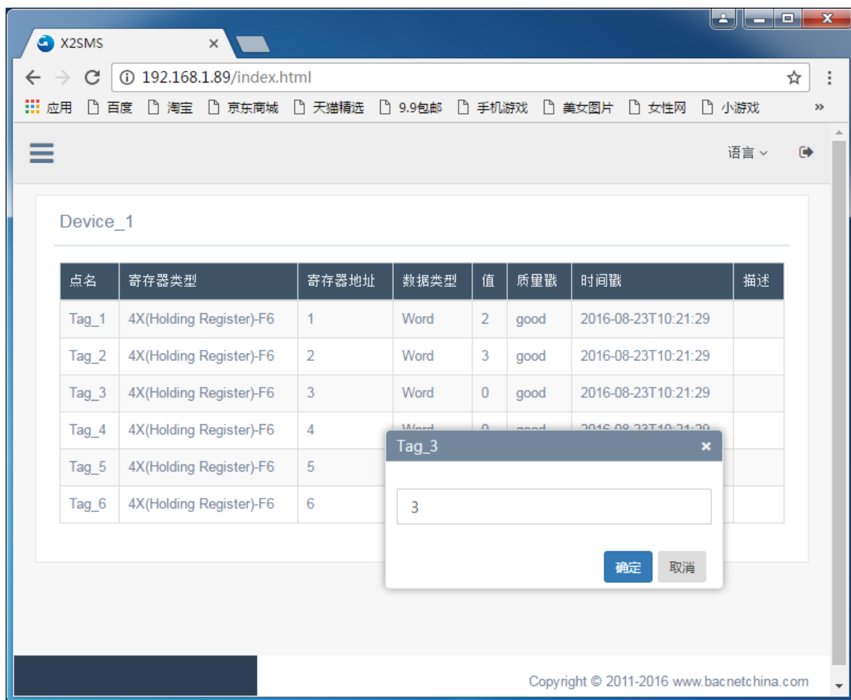
图 4-9-2 写值操作
