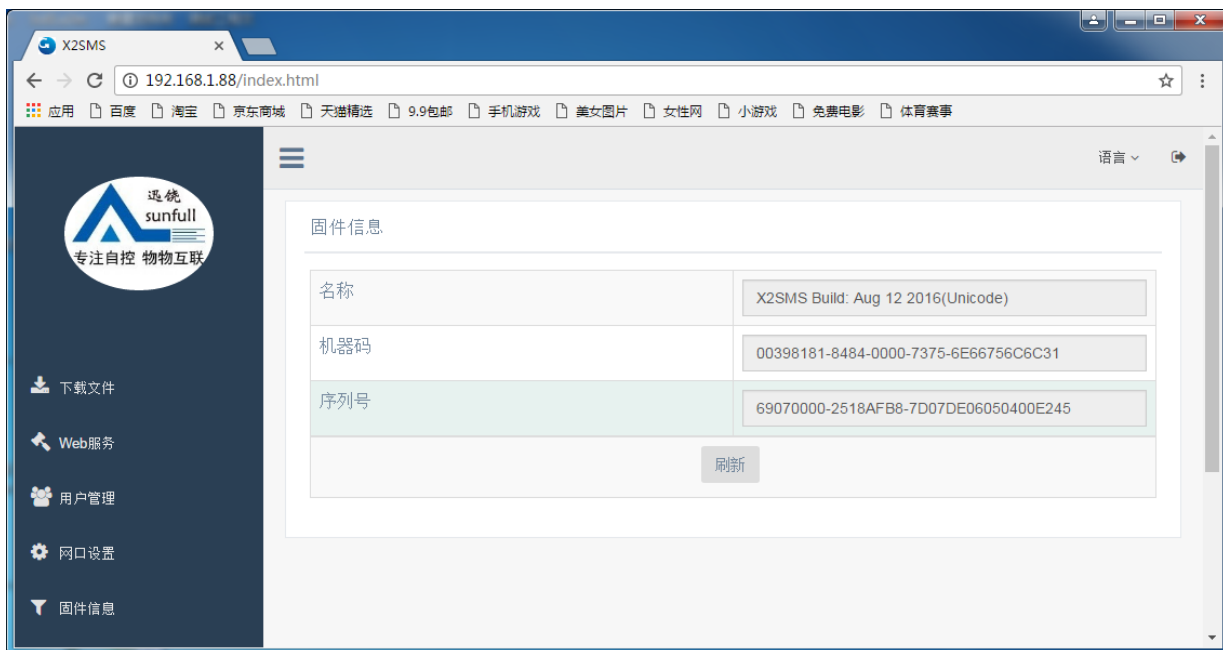
图 4-6-1 固件信息
