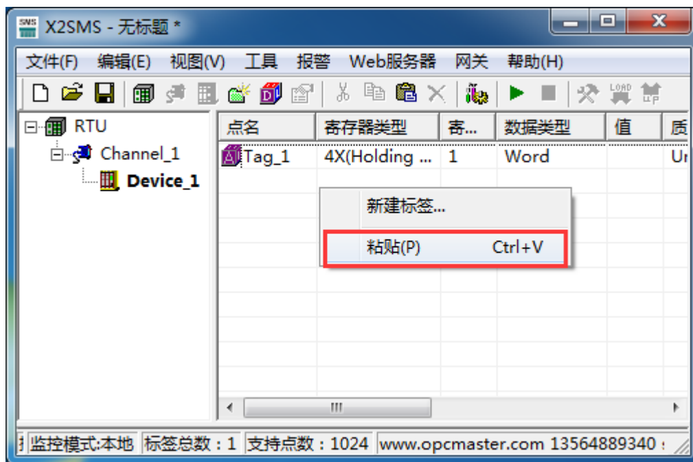
图 3-6-6 粘贴标签
