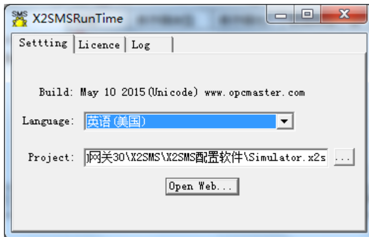
图 3-8-2 X2SMSRunTime 主界面
