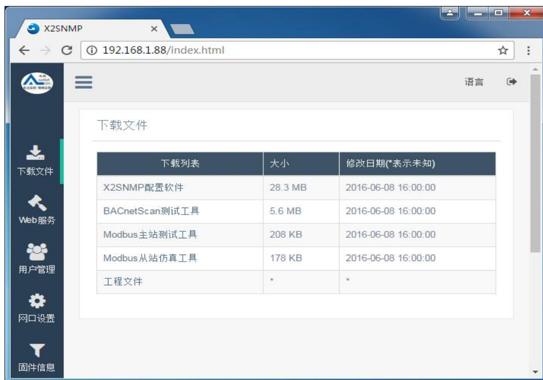
图 4-2-1 下载文件
